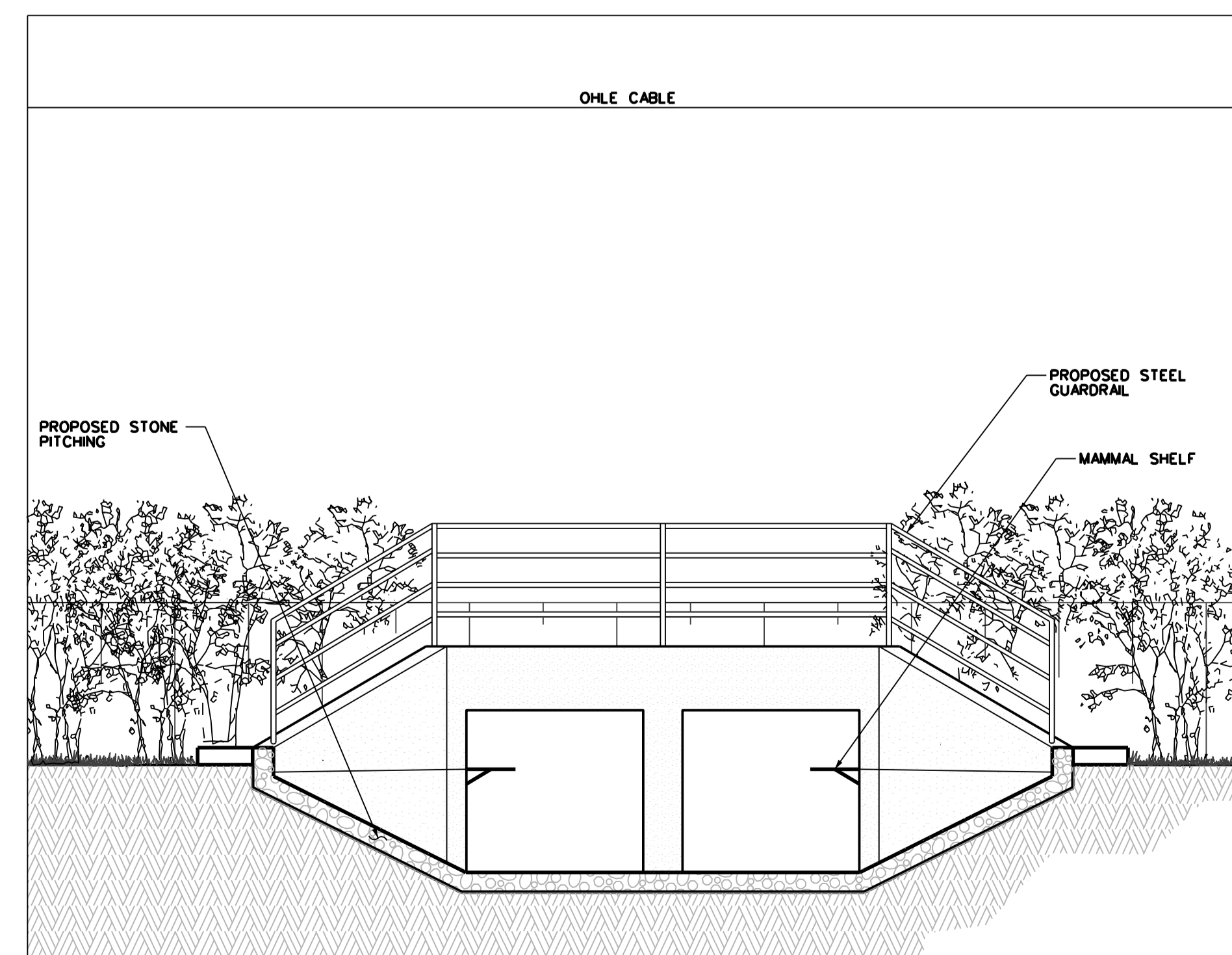
SECTIONAL ELEVATION B-B SCALE: 1:50
