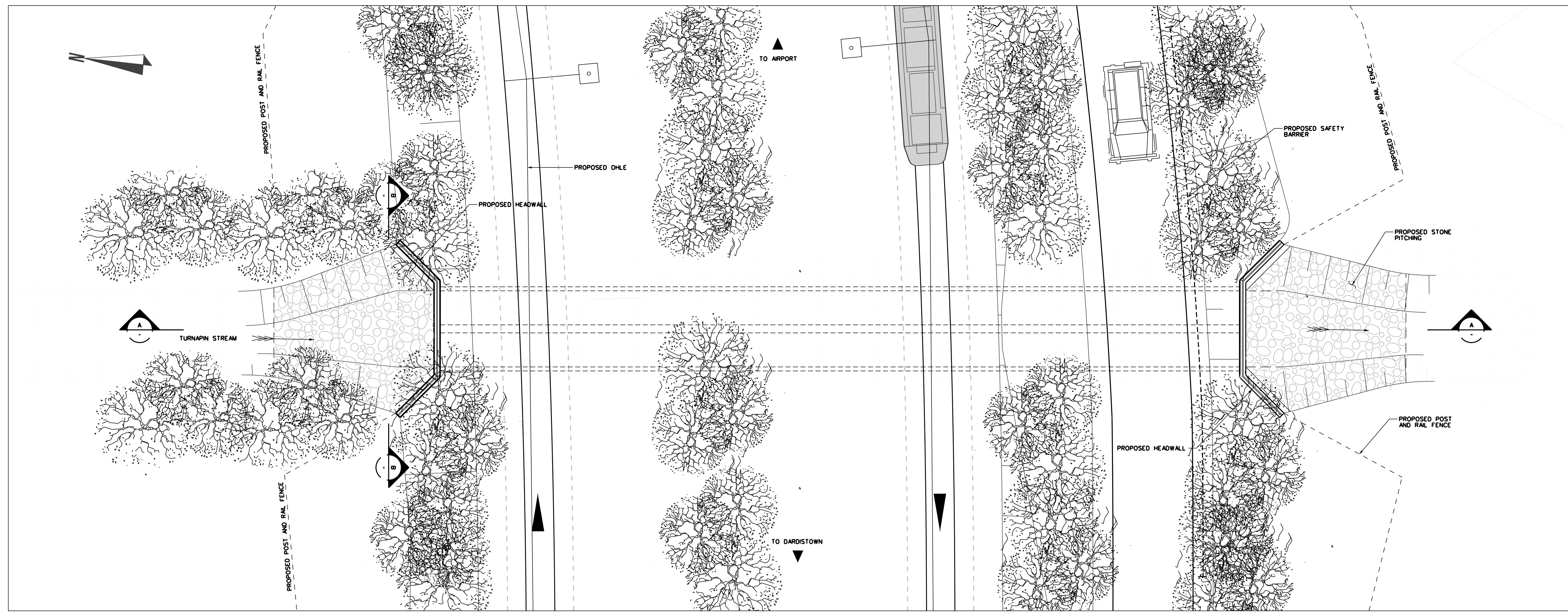
PLAN SCALE: 1:100
